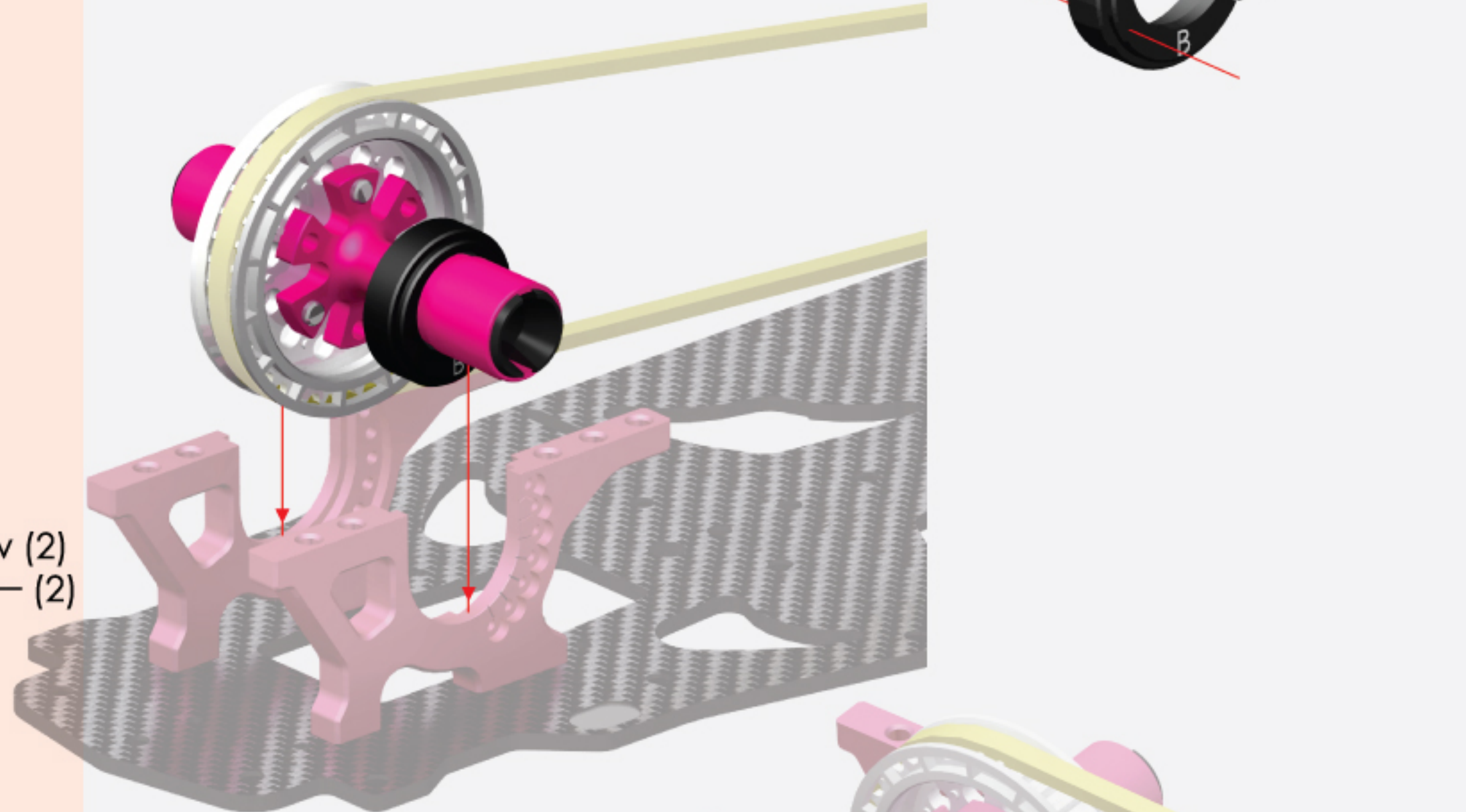
Bearing Holder - A(1) ベアリングホルダー - A(1)
