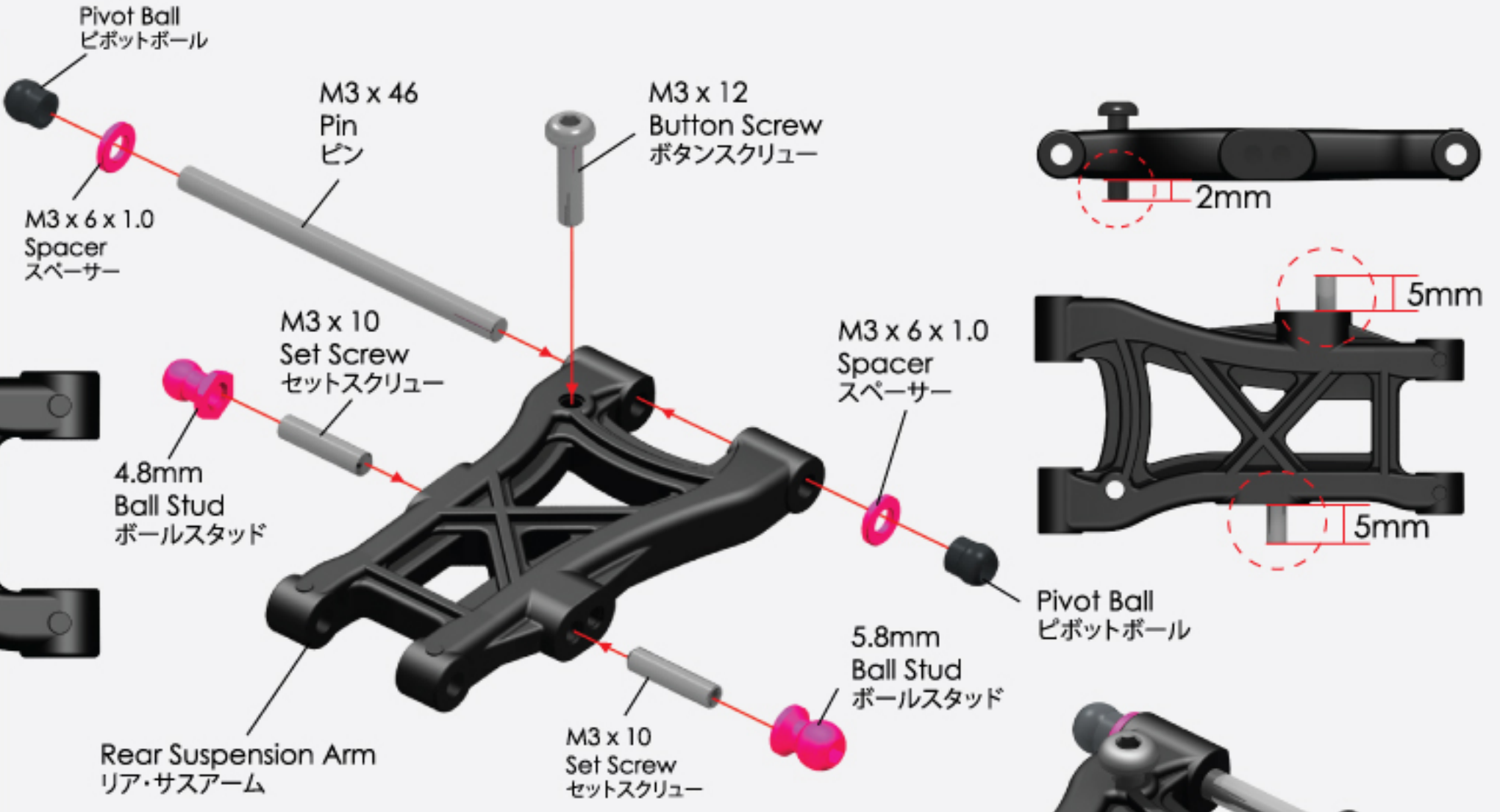
Rear Suspension Arm (2) リア・サスアーム (2)
